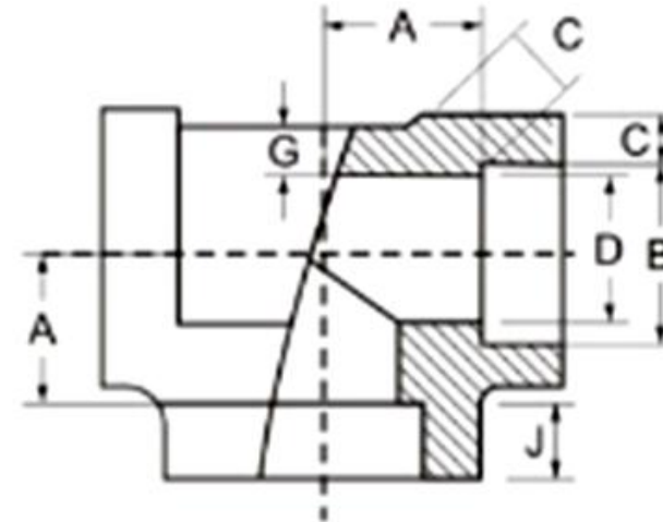
SW Tees
